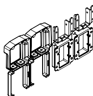
Supports intermédiaires
